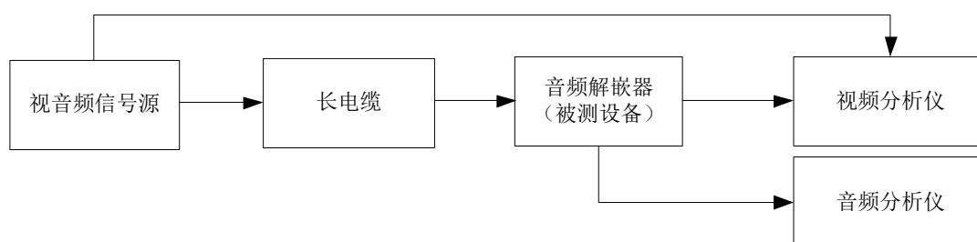
图2 SDI 输入接口最小接收灵敏度测量框图
