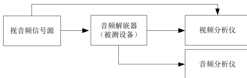
图1 SDI 输出接口、SDI 输入接口最大输入电压、视频通道特性、音视频相对延时、信号格式、数字音频输出接口、数字音频格式、音频通道特性测量框图
