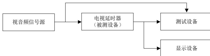
图12 延时测量框图
