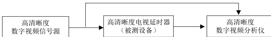
图8 SDI 输入接口最大输入电压测量框图
